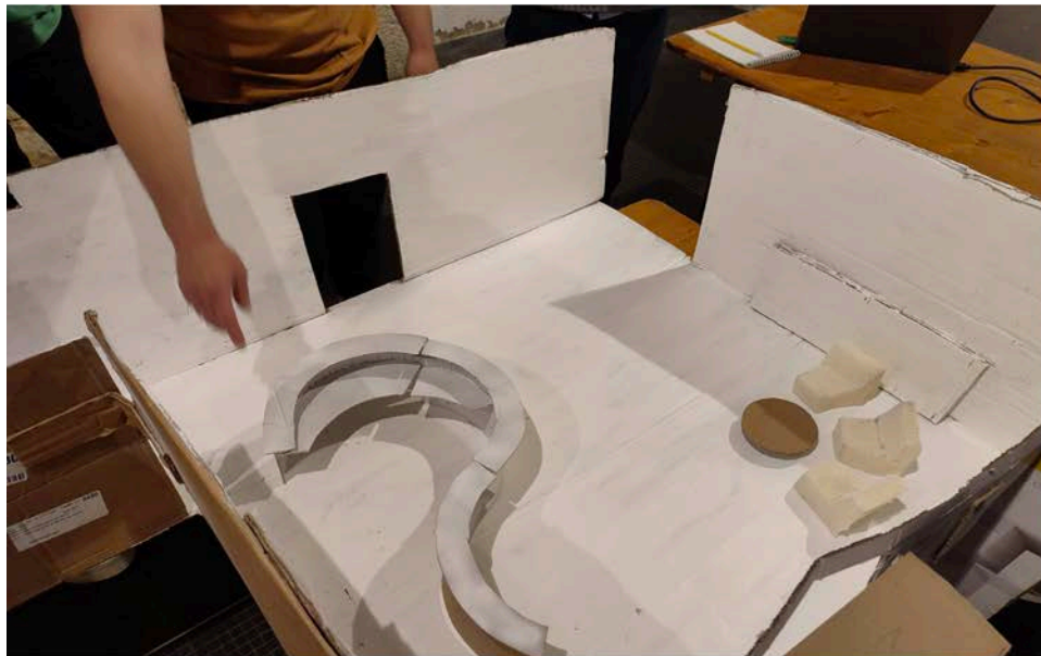
Prototypage en cours d'une assise pour l'espace détente du musée, réalisée à partir de mousse de tapis d'escalier
